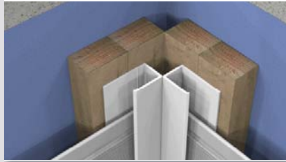
FC302E3 Universal Edge Trim
